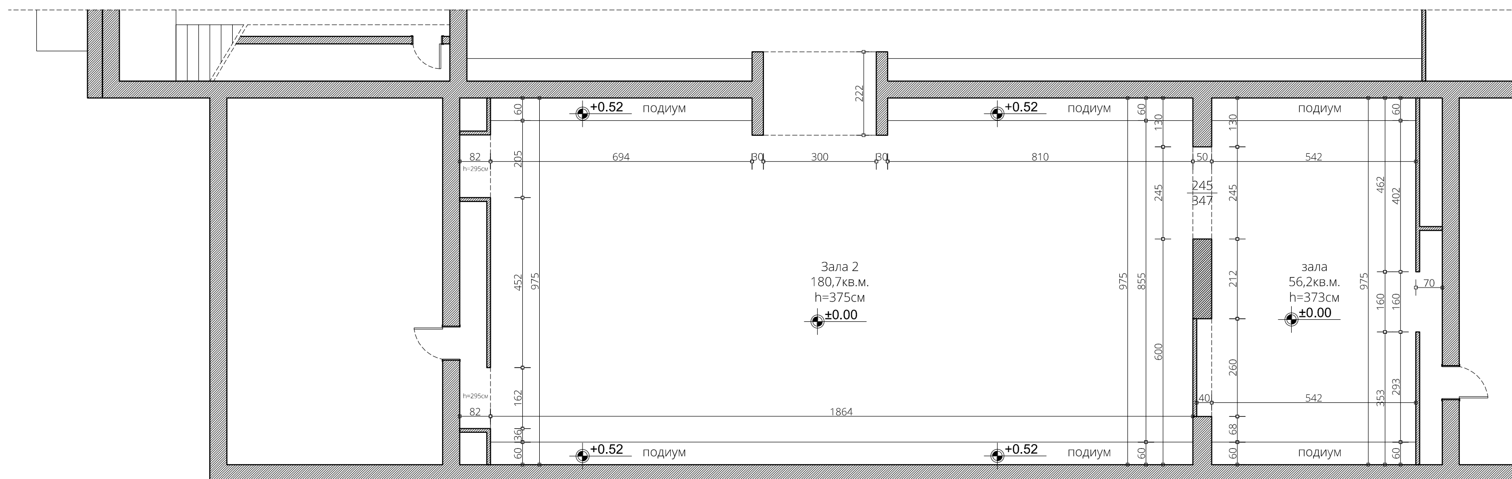
План Разпределение Партер Зала 2 М 1:100
