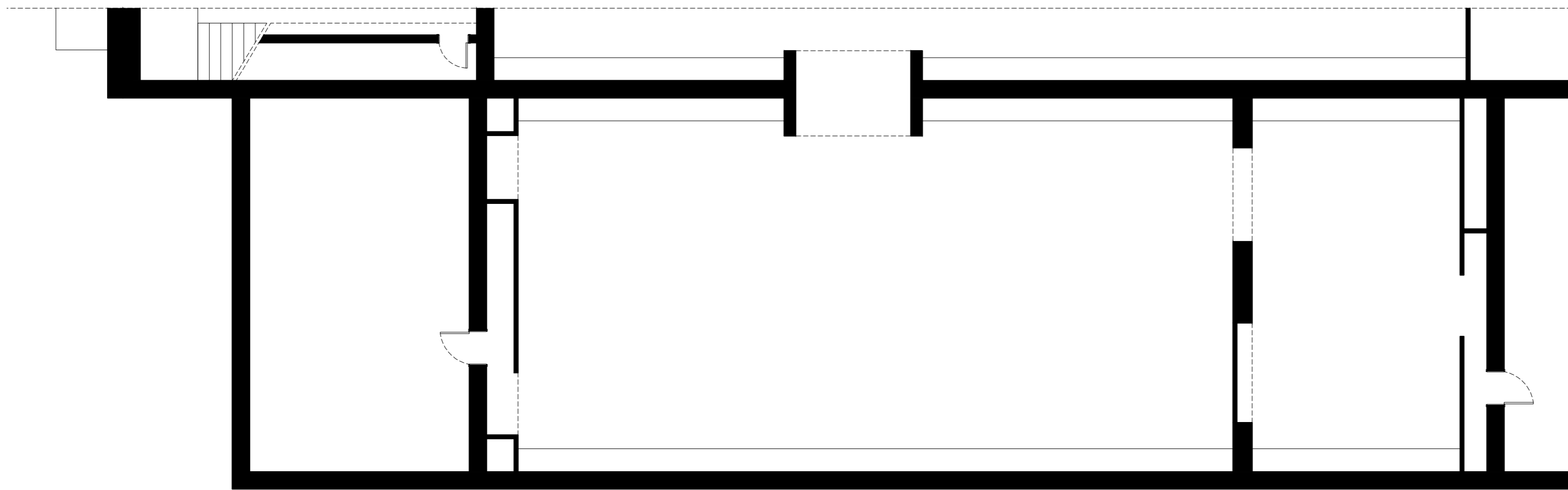
План Разделение Партер Зала 2 М 1:100
